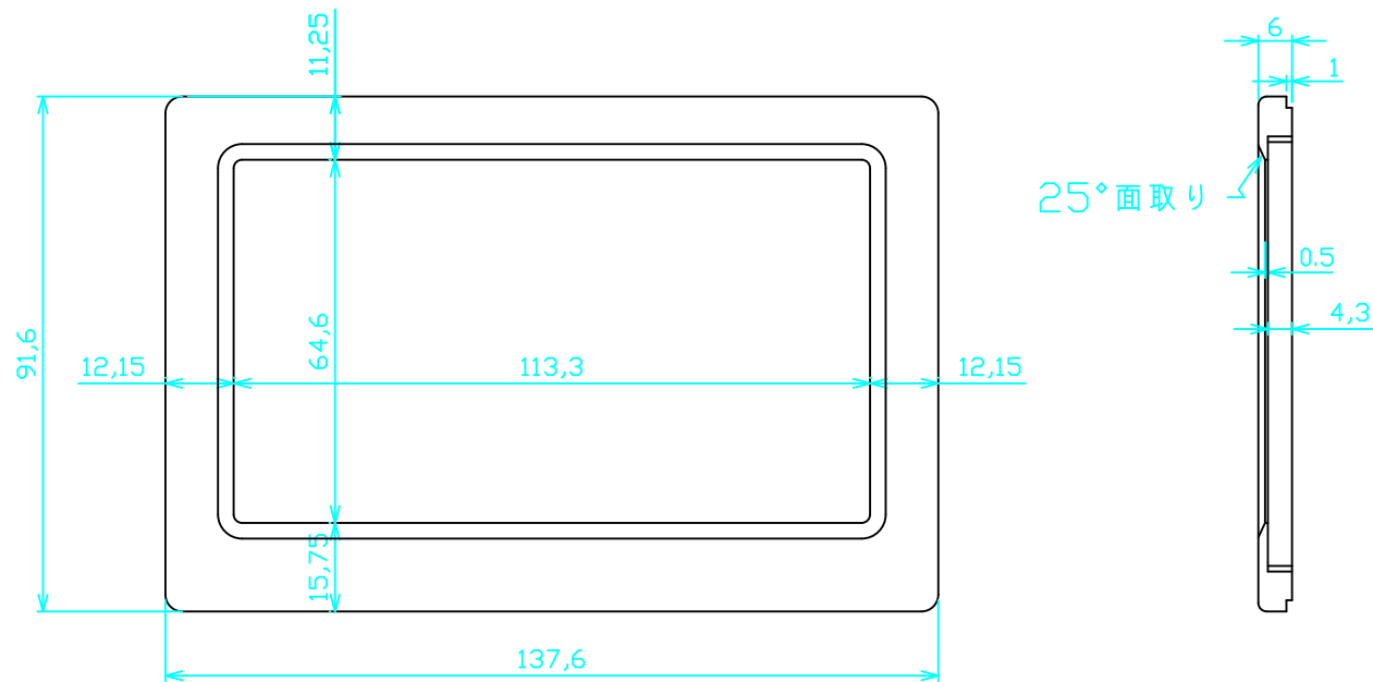
フレーム A5052 t6.0
