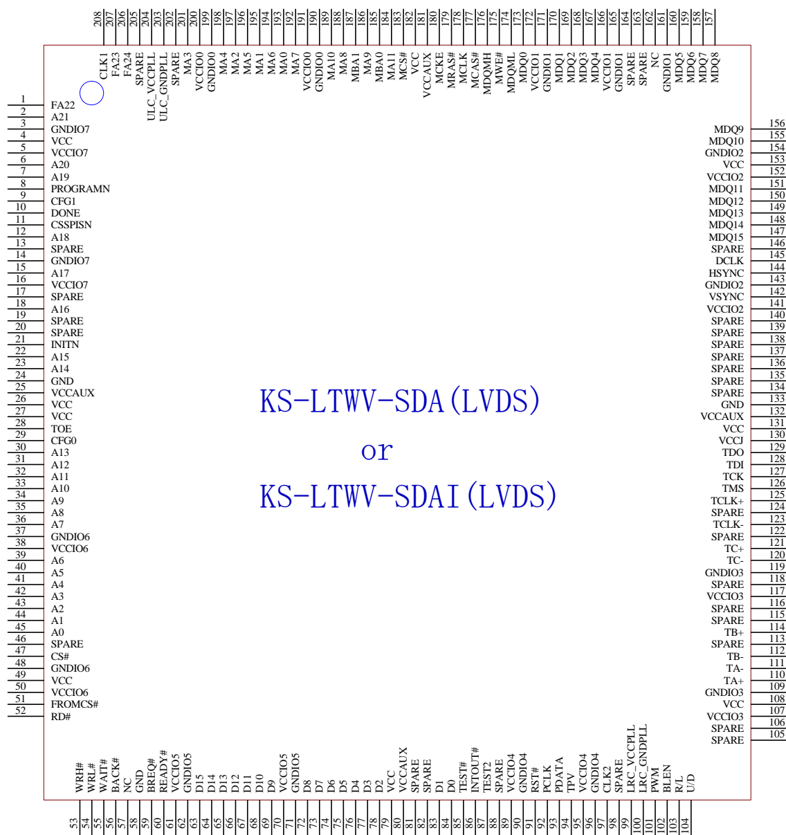
図) 端子配置図
